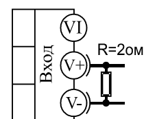
0...20 мА ТОКОВЫЙ вход
